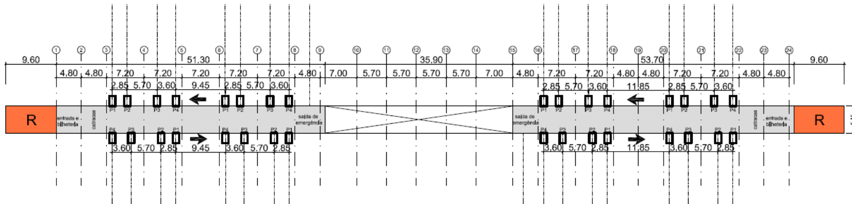
Figura Apêndice 5 - Croquis esquemático Estação Tipo 4 - Dois módulos Expresso e parador
